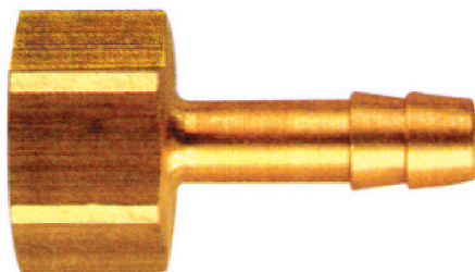
Female thread connection nippels-with hose tail - Brass Nippel mit Schlauchtülle Innengewinde Messing
