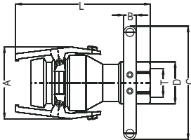
Self Sealing Female Threaded Coupler With Handle Verschlußkupplung mit Hand grill
