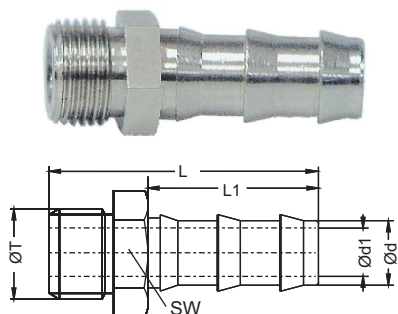
Push Lock Hose Nipple Gerade Nippel mit Schlauchklemmen
