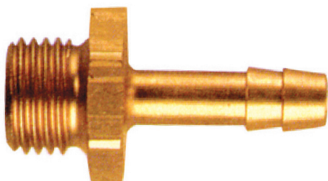
Male thread connection nippels-with hose tail - Brass Nippel mit Schlauchtülle Außengewinde Messing
